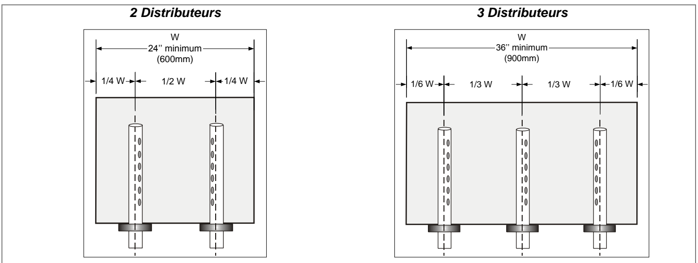
Illustration 15 - Distributeur 2" (51mm) diamètre emplacement: Conduits verticaux
