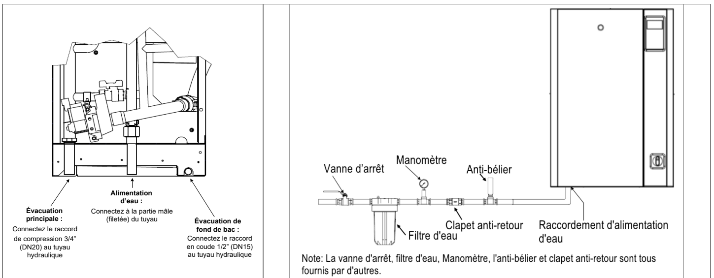
Illustration 31 - Raccordement d'alimentation et d'évacuation d'eau
